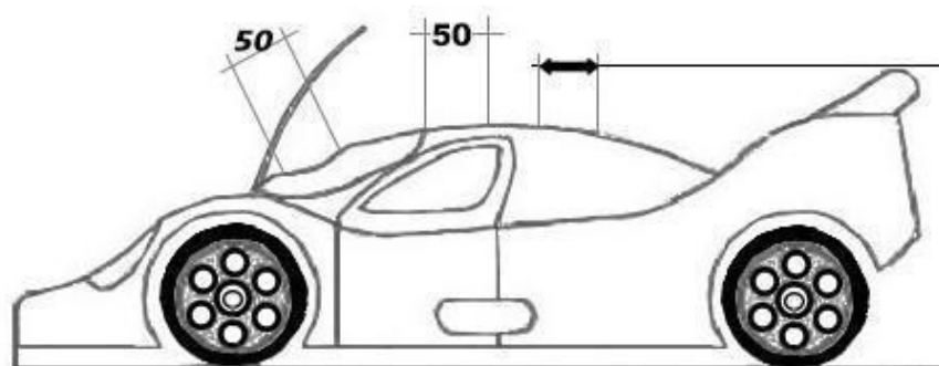
Figura 15 : Dimensioni max dei fori carrozzeria GT CARDANO Il completo di paraurti e bumper, dovrà rimanere compreso nelle dimensioni mass
