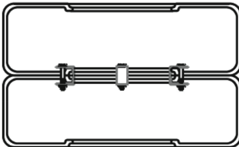
particolare assemblaggio
